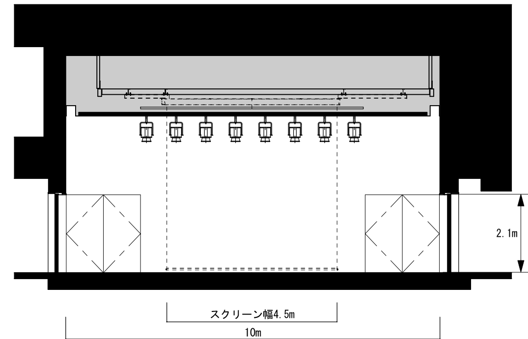
正面図
