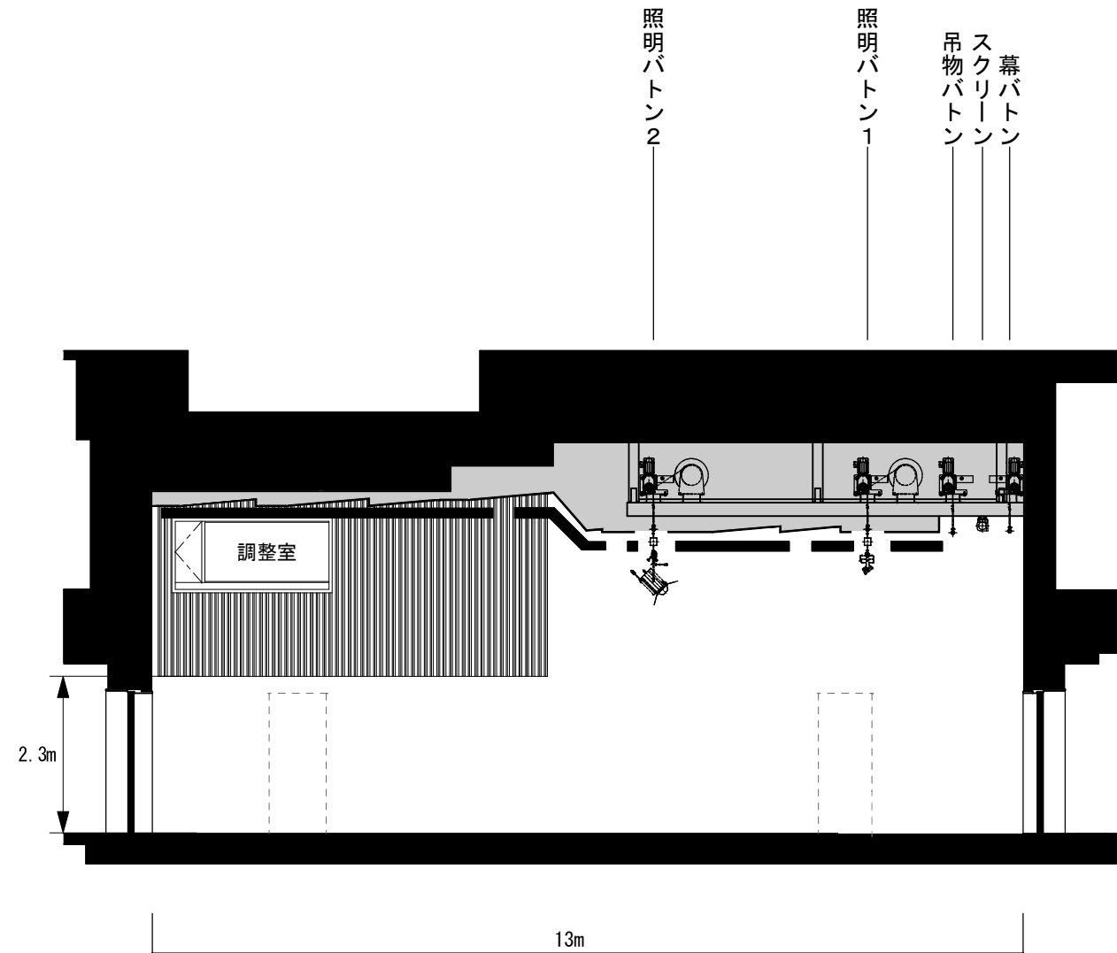
断面図
